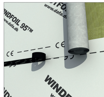
Her anvendes DAFA UV tape til overlap på DAFA Windfoil 95.
