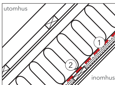
Principlösning . sluttande vägg i takkonstruktionen av trä.
