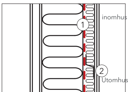
Principlösning - enkelt yttervägg i stål.
