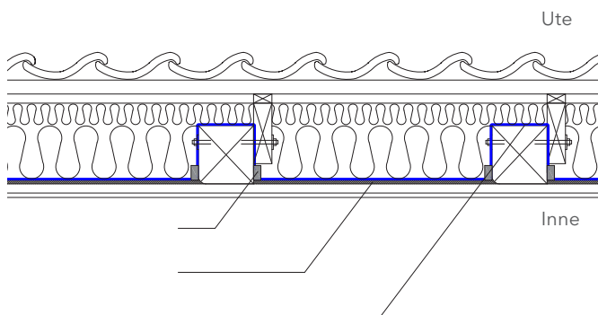
DAFA HiFoil läggs platt mot DAFA IsoBatt och över befintliga sparrar. Duken hålls fast mot sparrarna med DAFA klämlist.
