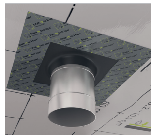
DAFA Hi-tack® rørmanchet anvendes til DAFA ExFoil og DAFA HiFoil damspærre.
