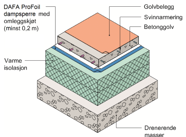
Fig. 3 DAFA ProFoil monterert i betonggolvpå grunnen.
