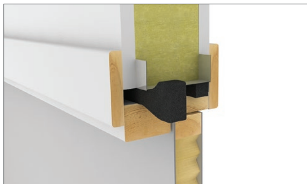
Lyddæmpning med illmod 600 fugebånd i dørkonstruktionen mellem stålprofilen og karmen.
