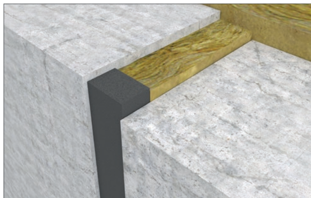
illmod 600 fugebånd anvendt til tætning ved samling af betonelementer.
