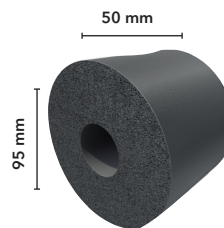
Type 95 95 mm x 50 mm Til 32 mm klemliste
