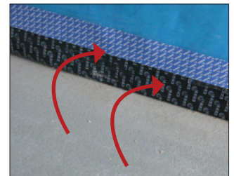
Det er vigtigt, at sokkel- og remfolien altid klæbes opad fast underlag
