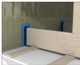
DAFA spærfodskrave monteret til etagebjælke
