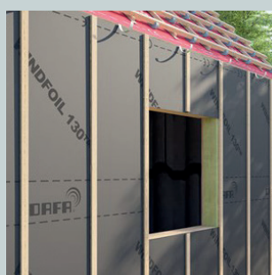
Vindskyddsduk
