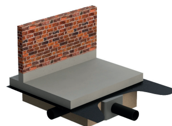
DAFA radonbrønd i et kapillarbrydende lag.
