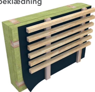
Åben facadebeklædning
