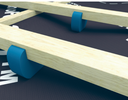
Et enkelt produkt med stor effekt. DAFA undertagsstrammer nedbringer montagetiden markant i forhold til traditionelle undertagsstrammere.
