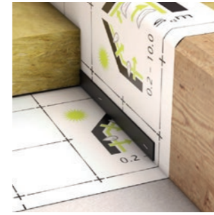
DAFA edge protection profiles
