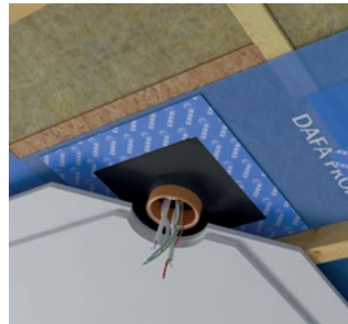
DAFA uni. cable collar 195
