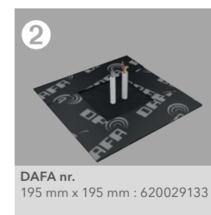
DAFA UV Radon kabelmanchett 195 – är en patenterad lösning som ger fullständigt säker tätning runt genomföringar för eldosor eller kablar.
