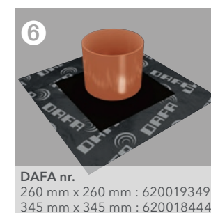
DAFA UV Radon rörmanchett – är en patenterad, lufttät lösning för tätning runt rörgenomföringar genom radonspärren.
